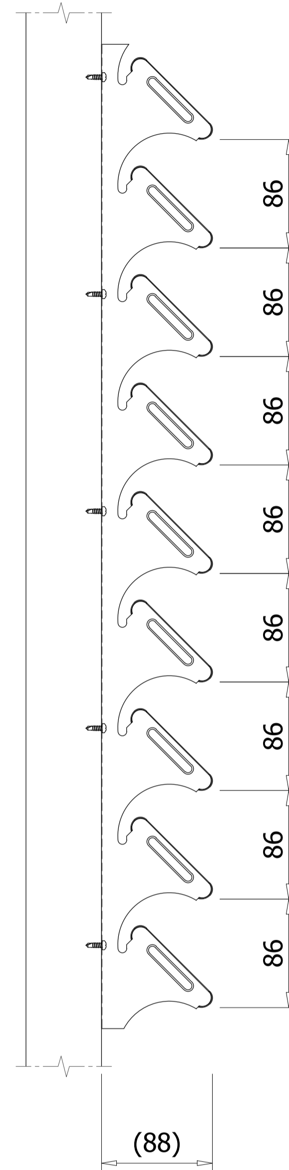
INSTALLATION DETAIL/ CHI TIẾT LẮP ĐẶT
