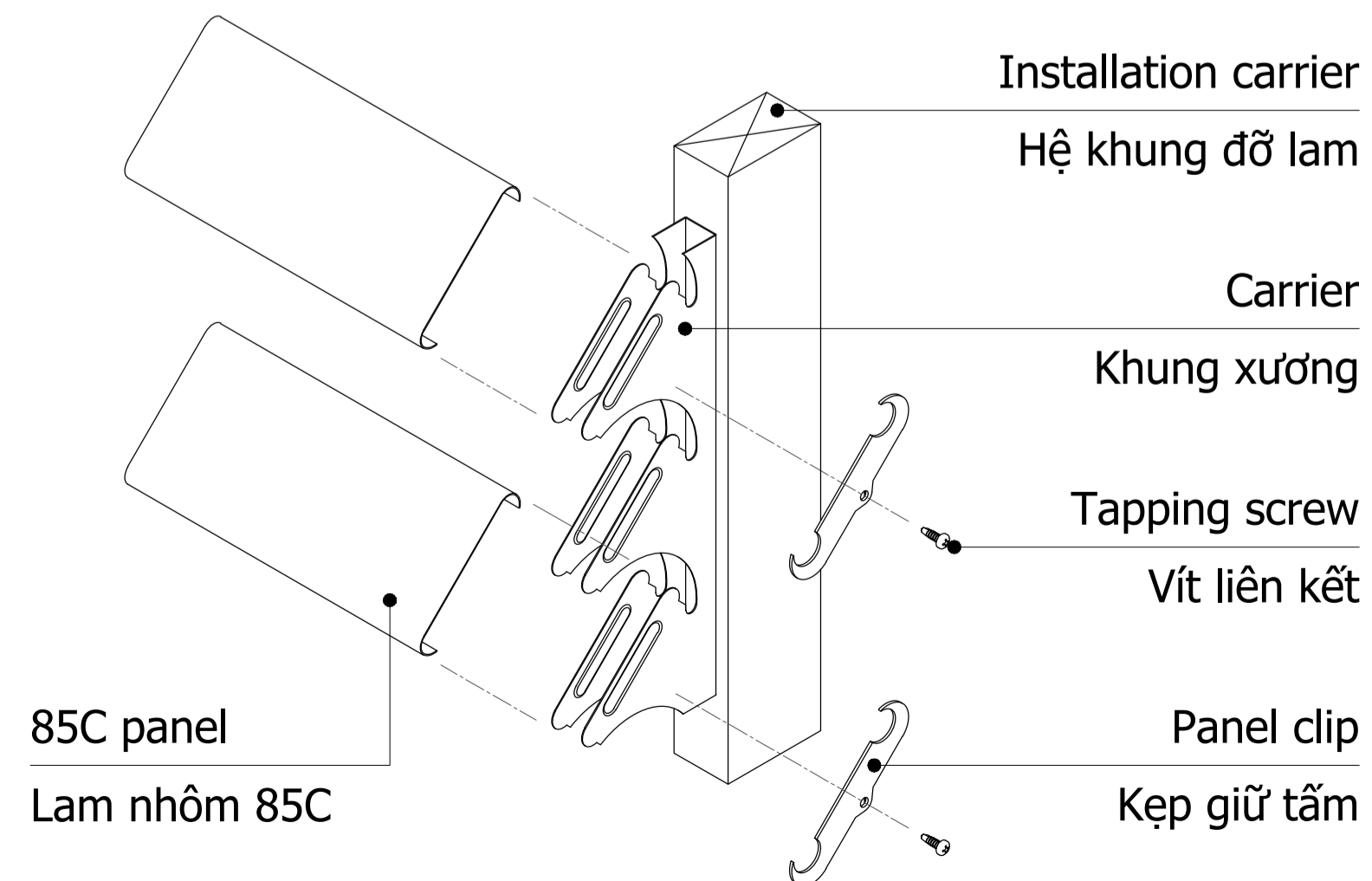
INSTALLATION DETAIL/ CHI TIẾT LẮP ĐẶT
